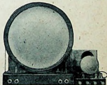
Fig. 6. Links een TV-chassis van dit jaar (819-lijnen, platte 63 cm beeldbuis, versnellingspanning 20 kV); daarnaast een chassis uit 1937 (455-lijnen, 18 cm-buis, 2 kV schermspanning)
